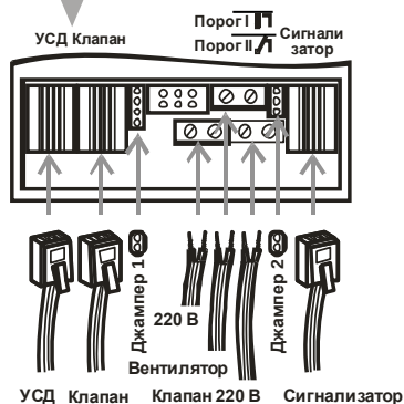
Рисунок 2 - Сигнализатор СИКЗ моноблочного исполнения
